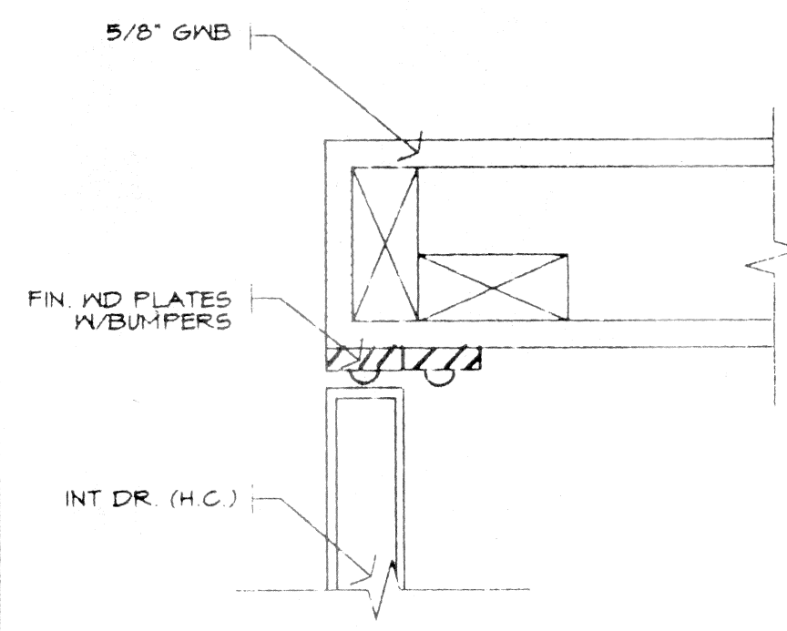
21 ALT. INT. DOOR JAMB TYP. @ 3" = 1'-0" 93184
